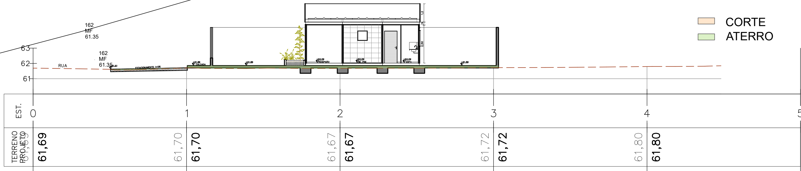
03 CORTES E ATERRO ESCALA 1/125
