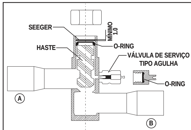
FIG. 28 - VÁLVULA DE SERVIÇO ABERTA
