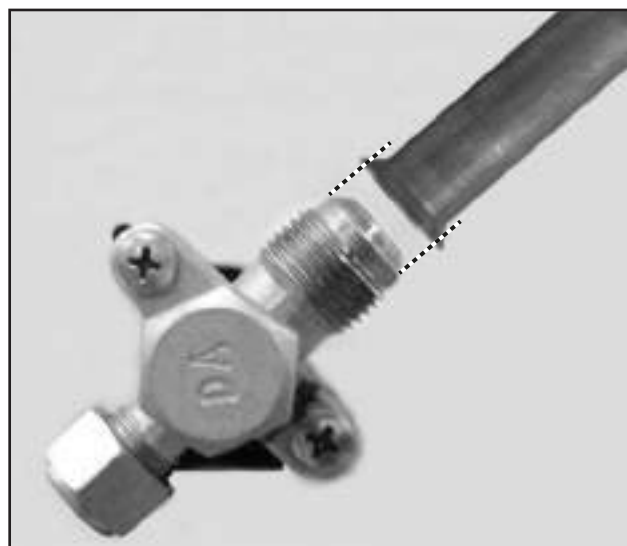
FIG. 32 - CONEXÃO NIPLE TUBO
