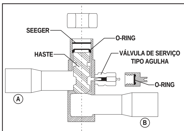
FIG. 27 - VÁLVULA DE SERVIÇO FECHADA
