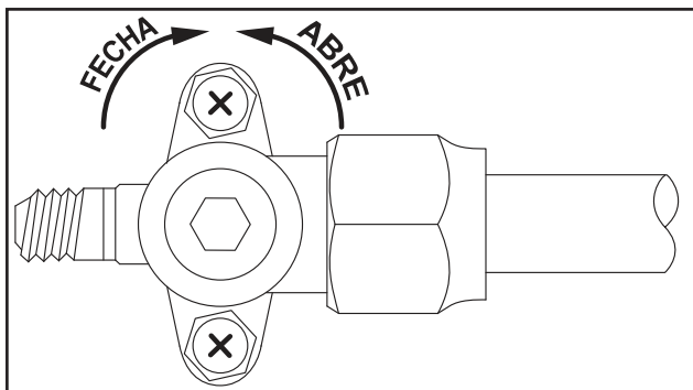
FIG. 26 - VÁLV. SERVIÇO SEM A PORCA DE PROTEÇÃO
