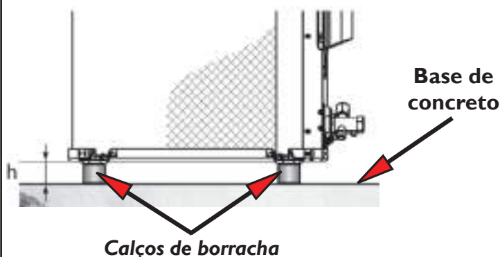
FIG. 4 - CALÇOS RECOMENDADOS PARA UNIDADES CONDENSADORAS
