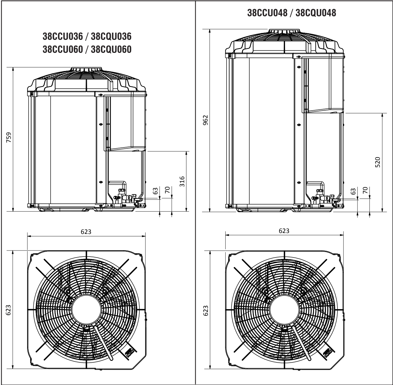
FIG. 13 - DIMENSIONAL UNIDADES CONDENSADORAS 38C
