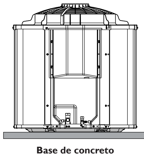
FIG. 4 - CALÇOS RECOMENDADOS PARA UNIDADES CONDENSADORAS
